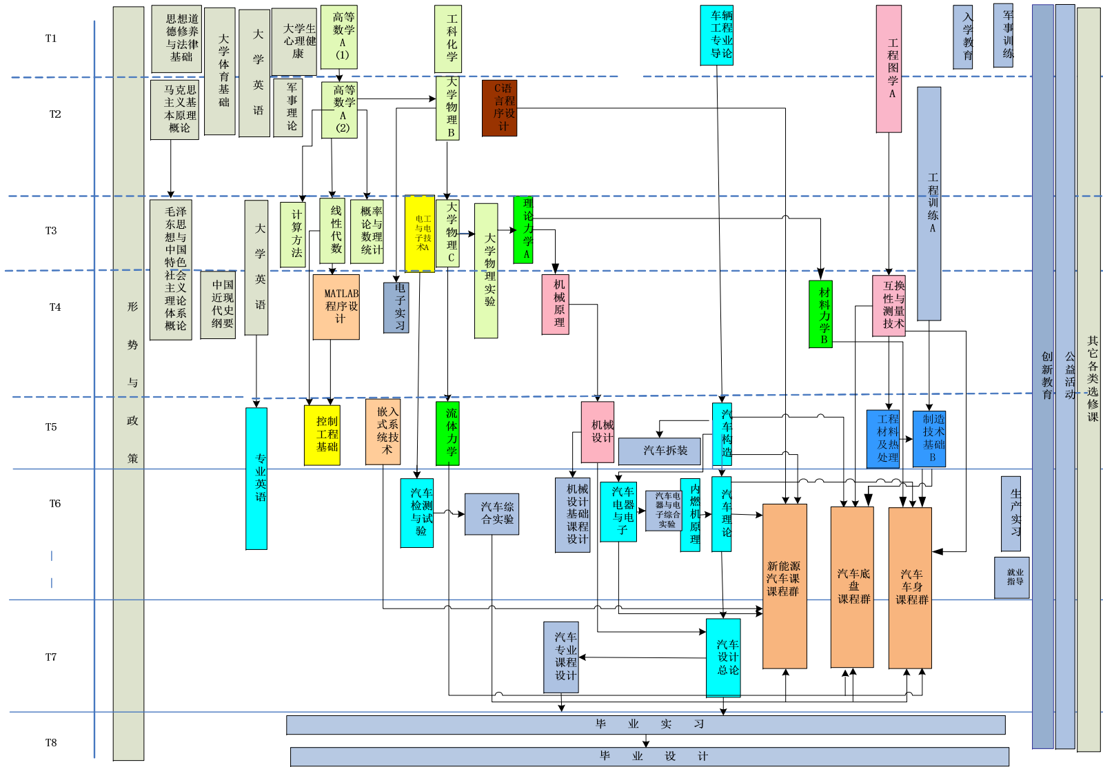
图 4 课程关系图
